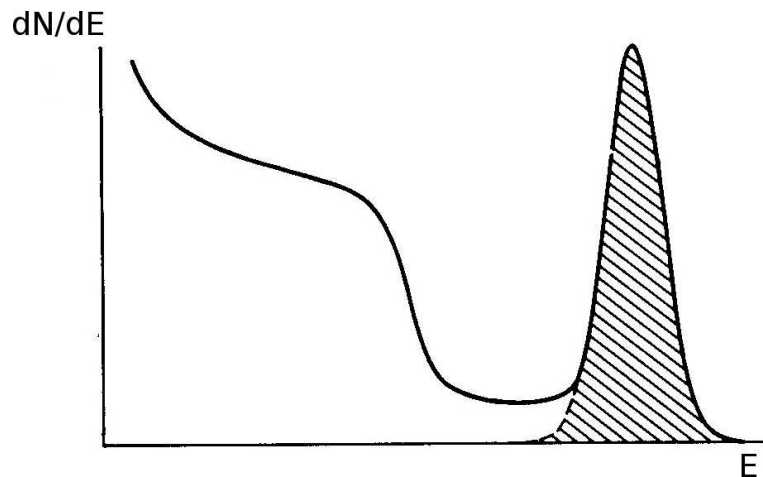
Widmo energetyczne
