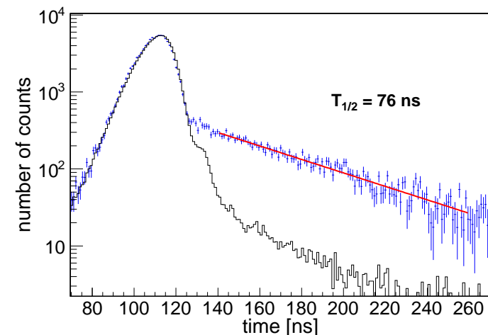
Widmo czasowe
