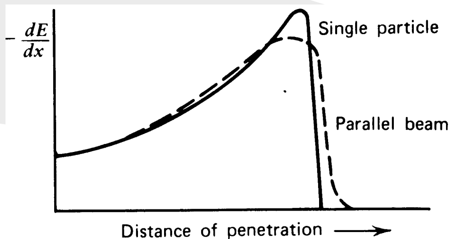
krzywa Bragga
