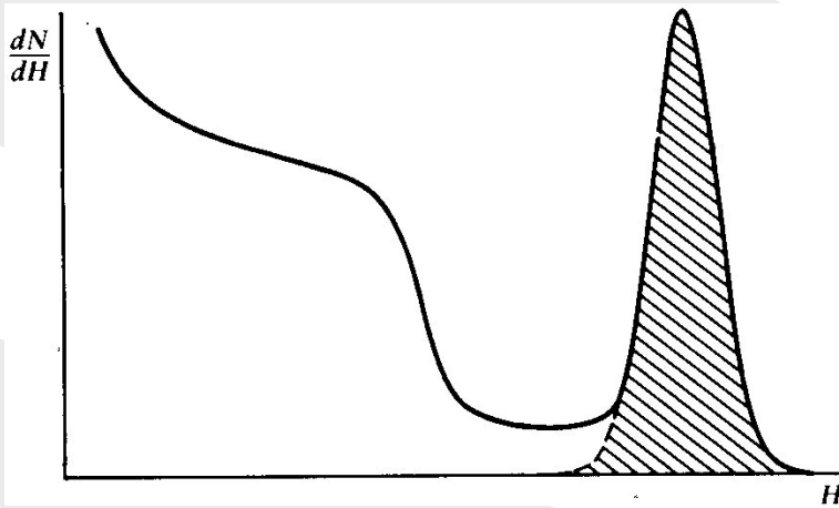
Widmo energetyczne
